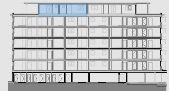
Coupe Générale
